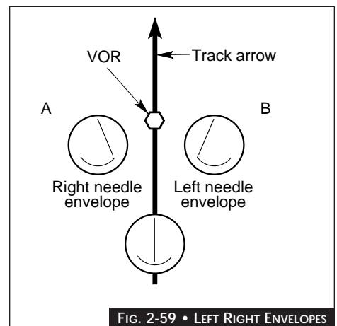
FIG. 2-59 • LEFT RIGHT ENVELOPES
