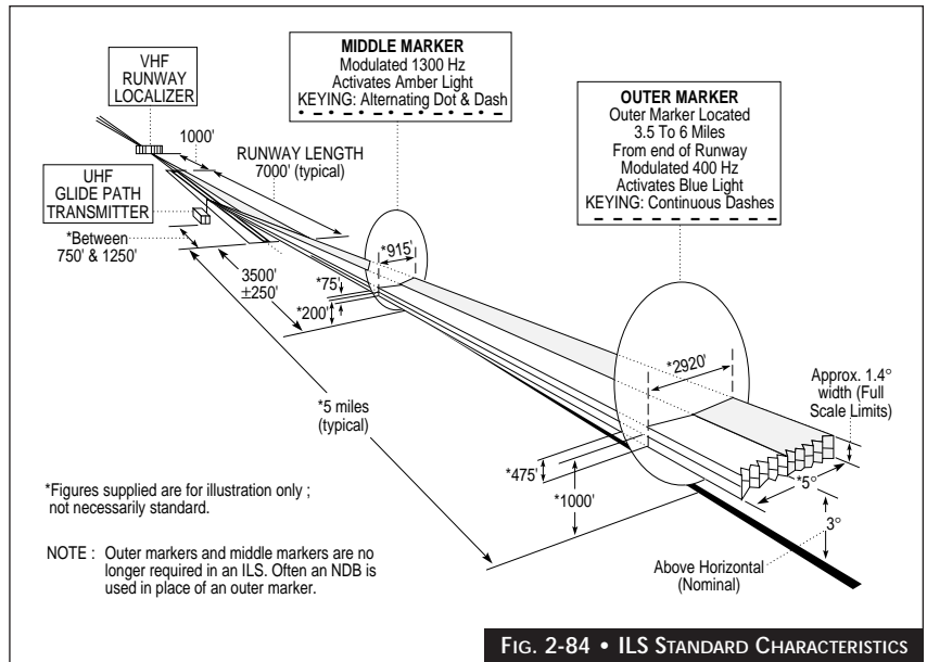
FIG. 2-84 • ILS STANDARD CHARACTERISTICS
