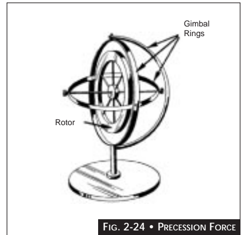
FIG. 2-24 • PRECESSION FORCE
